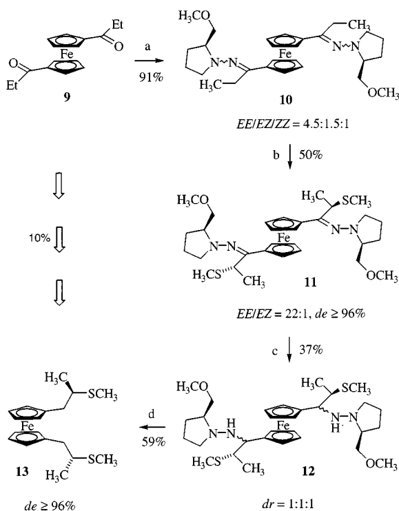
Scheme 5. Asymmetric synthesis of SUS ligand 13 : a) 4.0 equiv. SAMP/AlMe 3 , toluene, T ; b) 1) 2.5 equiv. LDA, 9.0 equiv. LiClO 4 , Et 2 O, room temp., 2) 3.0 equiv. (MeS) 2 , -100 °C; c) 8.0 equiv. catecholborane, CH 2 Cl 2 /Et 2 O, -50 °C to room temp.; d) TFA/NaBH 4 , CH 2 Cl 2 , 0 °C
